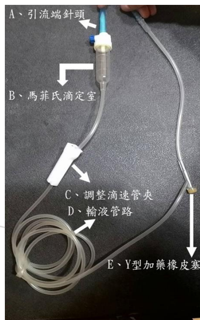
圖 1. 普通輸液套管結構圖
